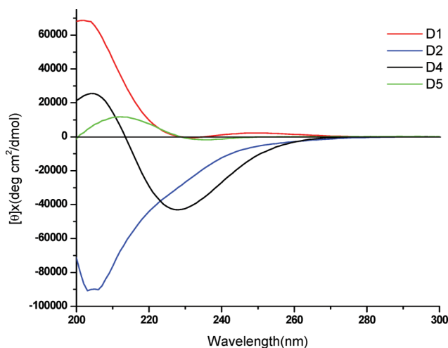
Fig. 6 Circular Dichroism spectra of dipeptides D1 , D2 , D4 and D5 in methanol.
